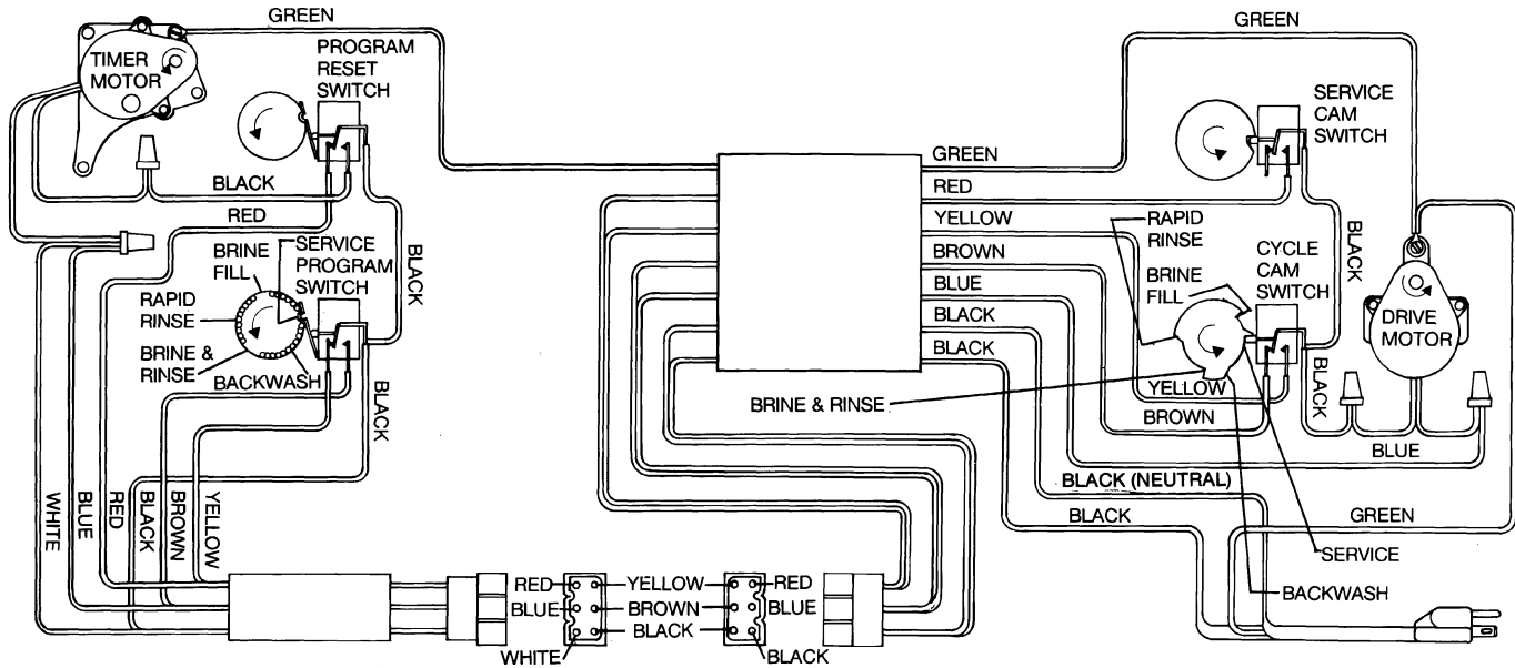
9000 WIRING DIAGRAM
