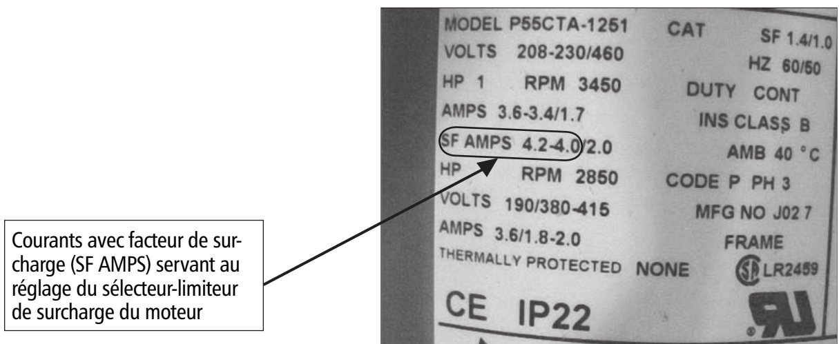
Figure 5 — Courant avec facteur de surcharge (SF AMPS) sur plaque signalétique de moteur type
